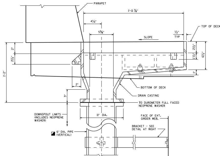
SECTION A1
