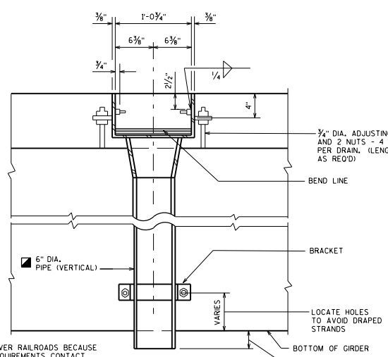
SECTION A2
