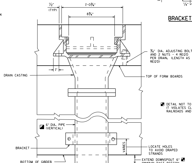
SECTION A2
