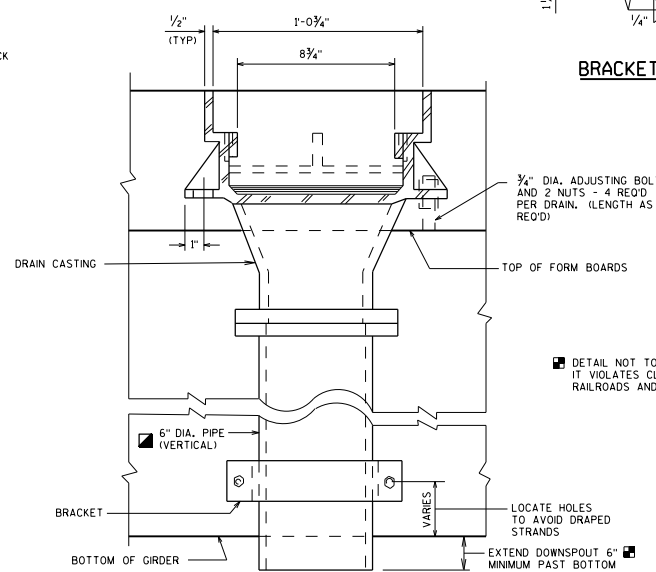
SECTION A2
