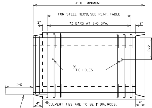
LONGITUDINAL SECTION
