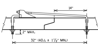
CANOPY TIE
